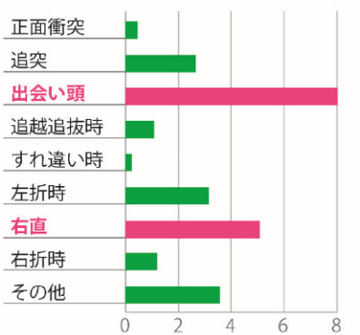
図1：事故類型別二輪車運転者の死傷者数 (第1第2当事者合計、2015～2019年)
